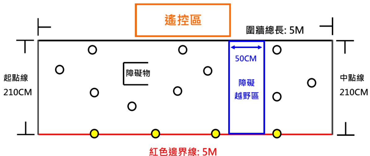
[圖一] 比賽場地示意圖
